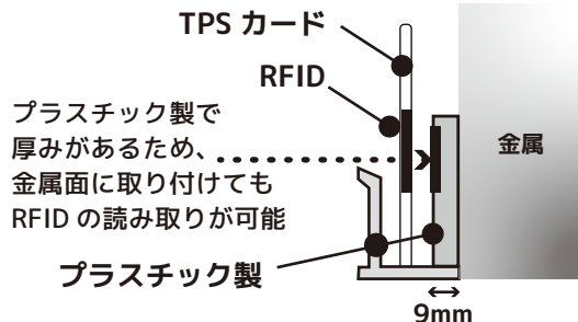
【カードを差した時の断面図】
